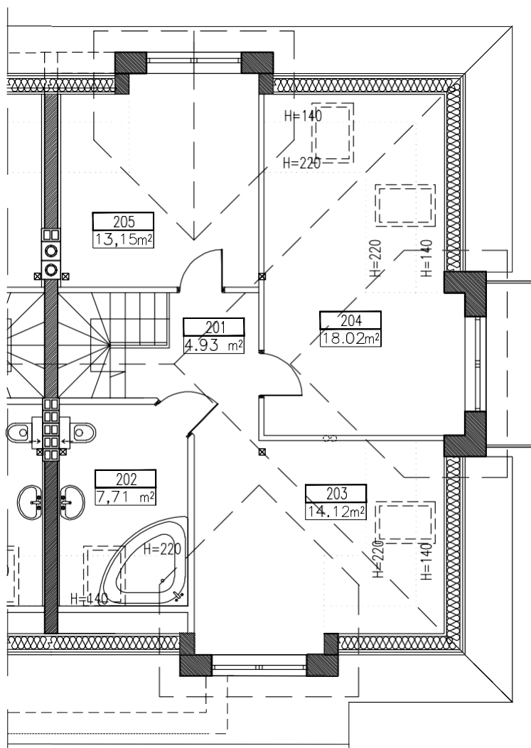
RZUT PODDASZA
